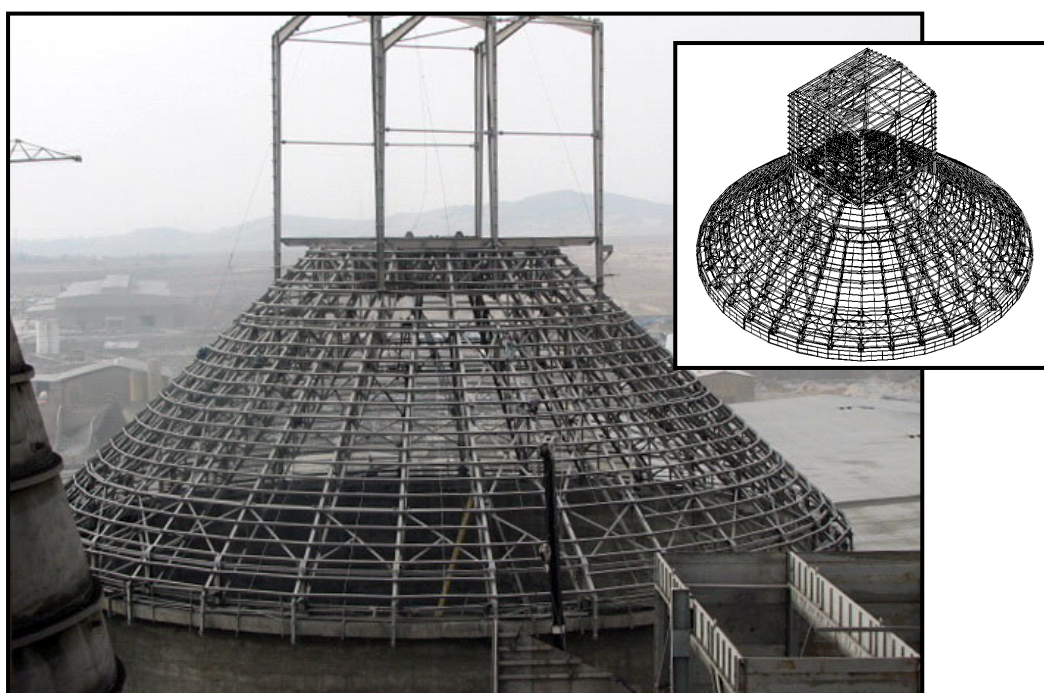
سازه سيلوی کليکر به ظرفيت ۸۰۰۰۰ تن به قطر ۴۶ متر و ارتفاع ۳۴ متر (کارخانه سيمان آبيک)
