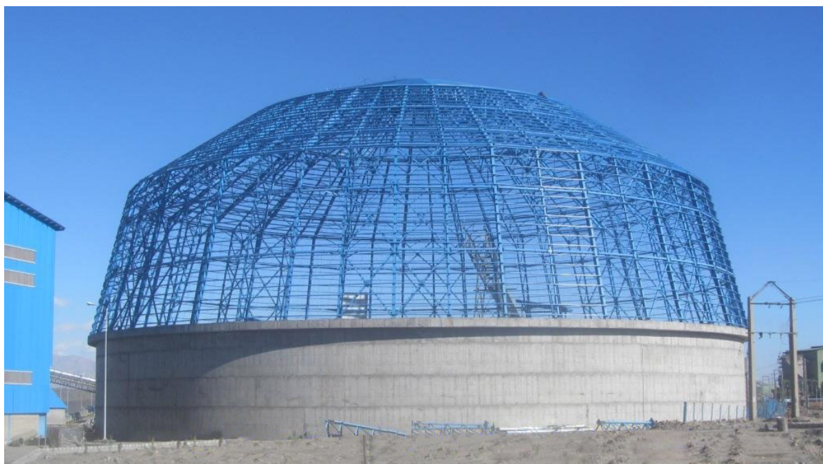
Stock Pile پروژه پلی کام (گل گهر سیرجان)
